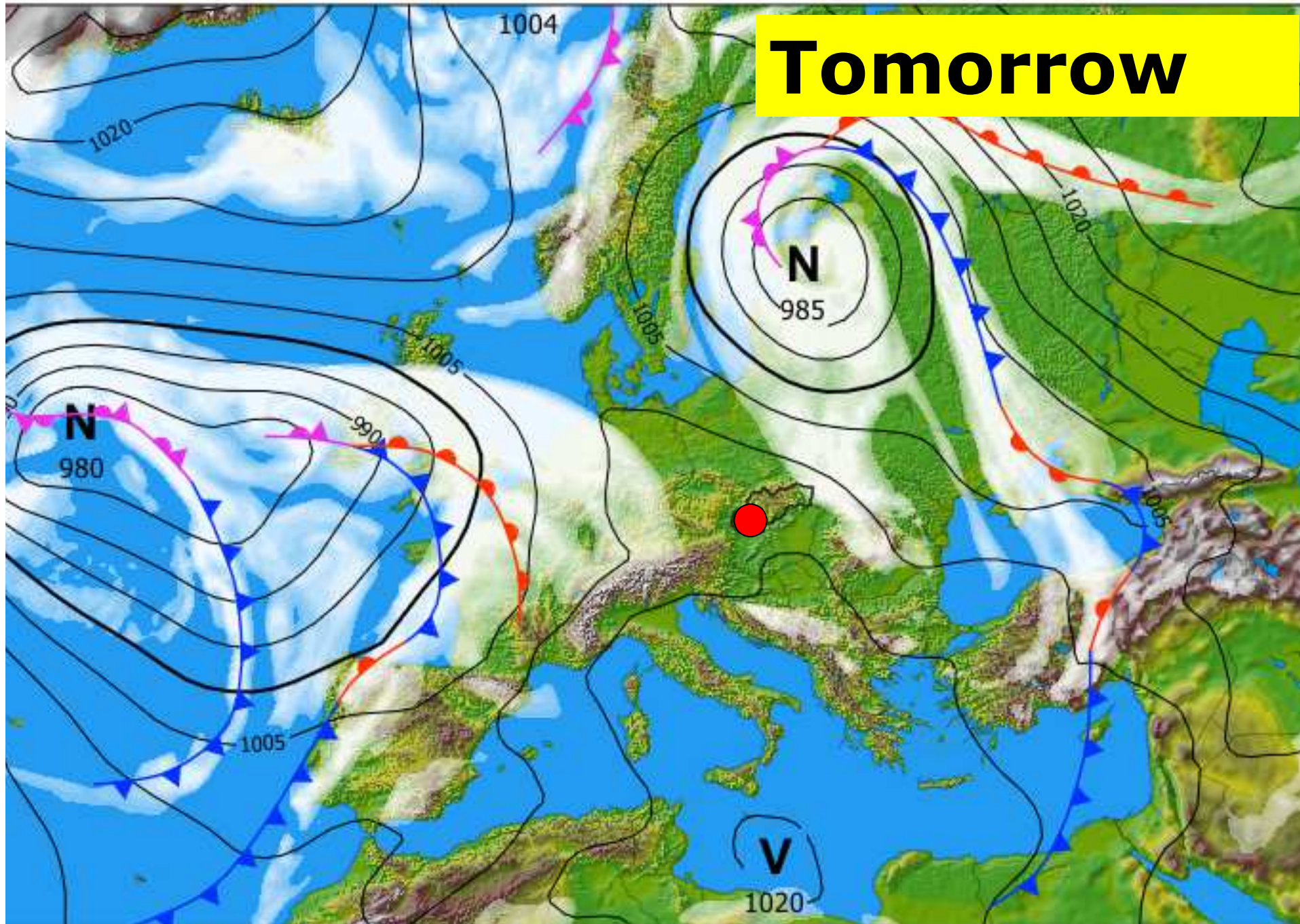
(c) SHMÚ - Prízemné tlakové pole - pondelok 02.04.2018 12:00 UTC
