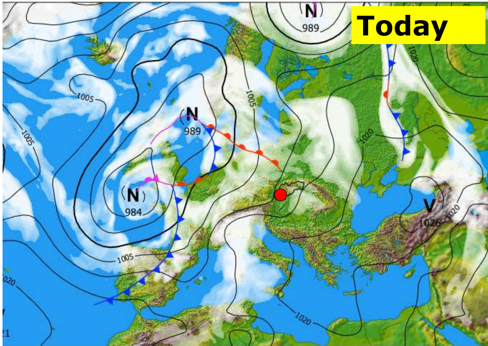
(c) SHMÚ - Prízemné tlakové pole - streda 04.04.2018 00:00 UTC
